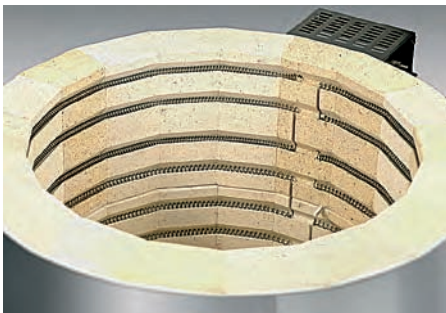
Ofen Innenansicht
